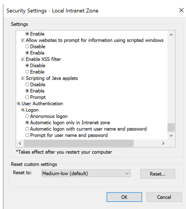
Рисунок 6 – Настройки Windows для входа через сеанс ОС (продолжение)
