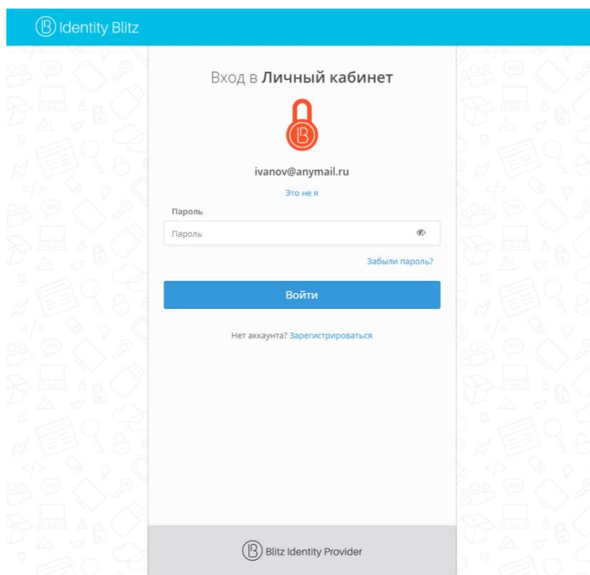
Рисунок 2 – Вид экрана входа с сохраненной учетной записью
