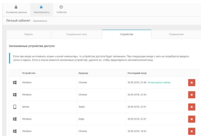
Рисунок 23 – Просмотр и управление списком запомненных устройств
